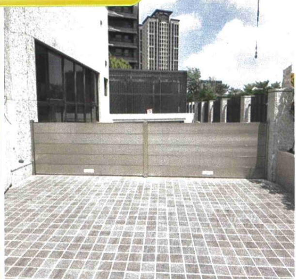
車道組合式防水閘門
